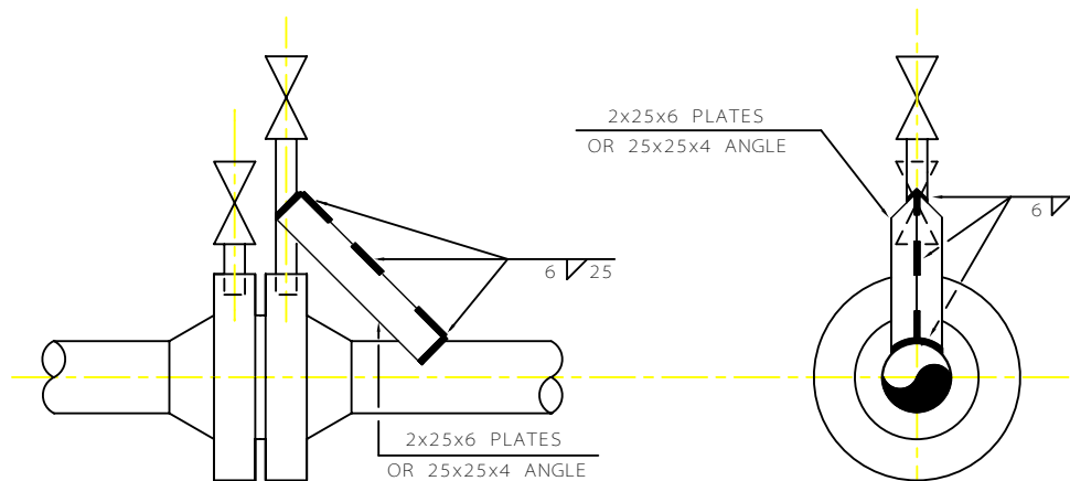
No.3 LONGITUDINAL BRACE
