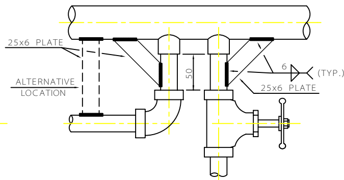
No.2 LONGITUDINAL BRACE
